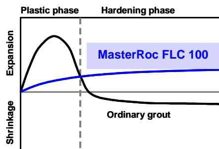
Схема действия MasterRoc FLC 100 при отрыве стального анкера
